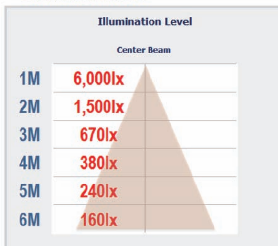
Conical Illumination 照度分布図
